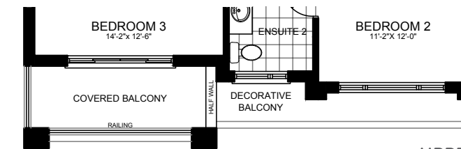
ELEV. C
