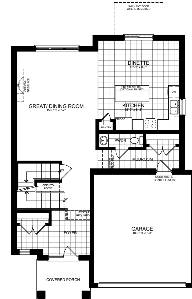
ELEV. A & B
