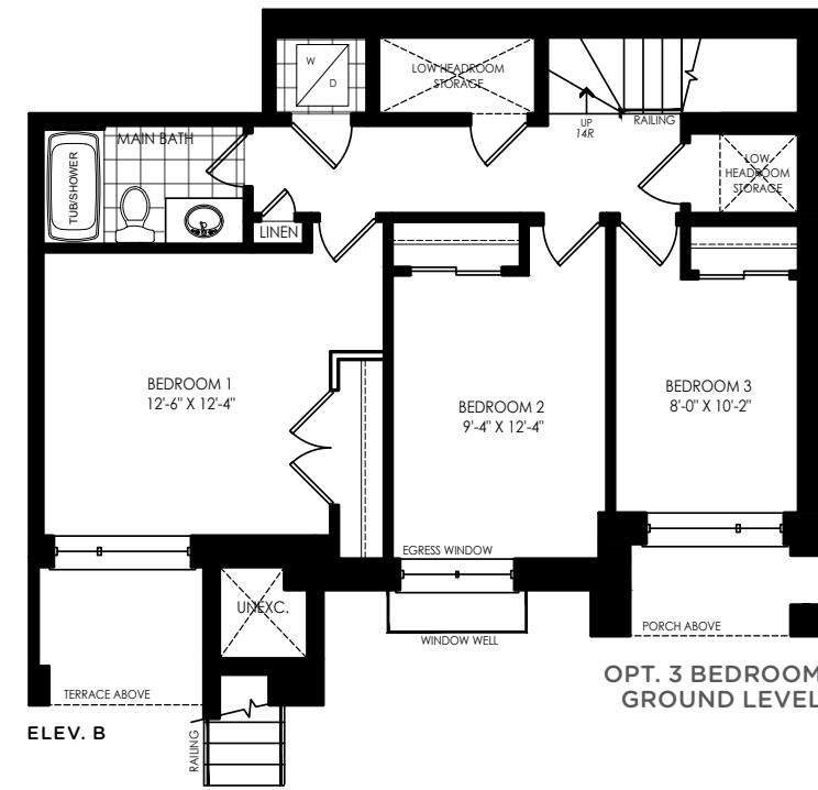
ELEV. B
