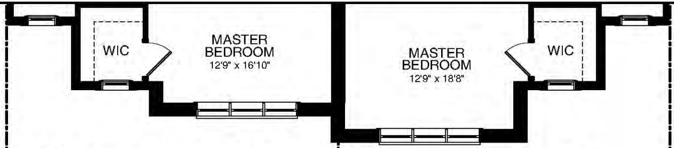
SECOND FLOOR ELEV. D1
